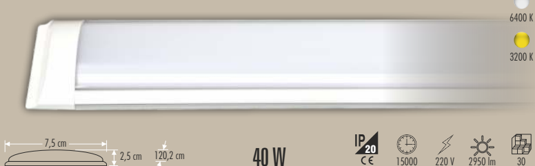
CT-2476 GOLD YATAY BANT ARMATÜR DOUBLE ALÜMİNYUM KASA
